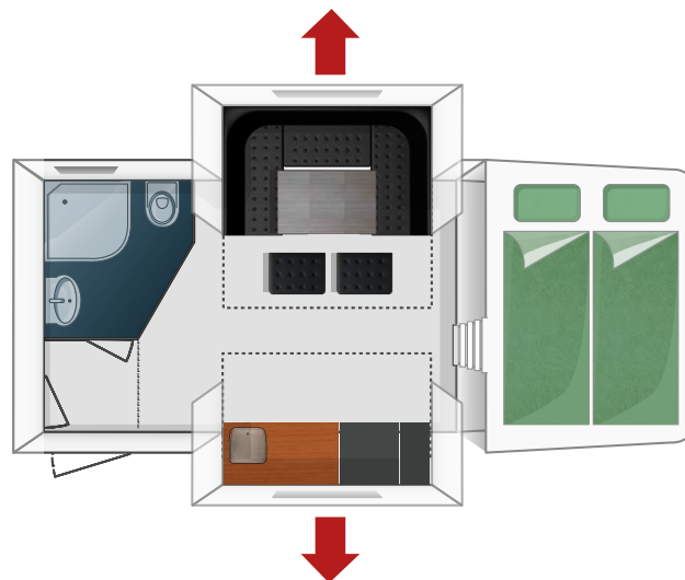
DOPPEL POP-OUT SEITLICH / Double pop-out at side
