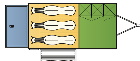
Big Trailer L3 (6,5 t) mit begehbare Sattelkammer Big Trailer L3 (6.5 t) with walk-in tack room
