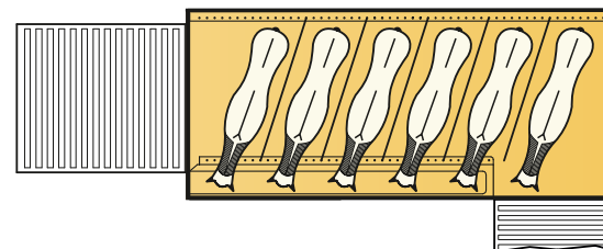
Pferderaum mit durchgehenden L-Trennwänden (siehe Seite 17) und seitlich integrierter Sattelkammer mit durchgehendem Futtertrog Horse compartment with full L-partitions (turn to page 17) and tack room integrated at the side with full-length feed trough
