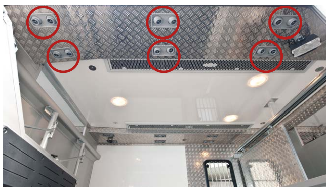
Lüftungsauslässe , mit einzeln einstellbaren Düsen Ventilation vents with individually adjustable jets
