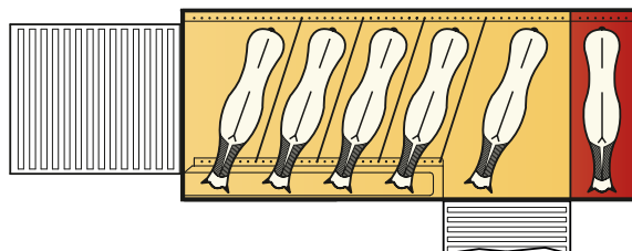
Pferderaum mit durchgehenden L-Trennwänden (siehe Seite 17) und seitlich integrierter Sattelkammer mit durchgehendem Futtertrog und Einzelstellplatz (Hengstbox) Horse compartment with full L-partitions (turn to page 17) and tack room integrated at the side with full-length feeding trough and separate single box (stallion box)
